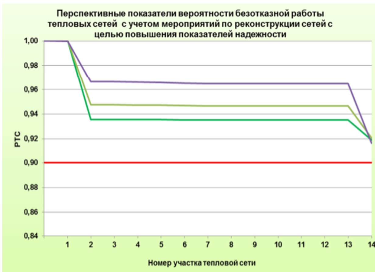
Рисунок 1.11 Вероятность безотказной работы тепловых сетей от Архангельской ТЭЦ до потребителя ИП Зеленин с учетом проведения предложенных мероприятий
