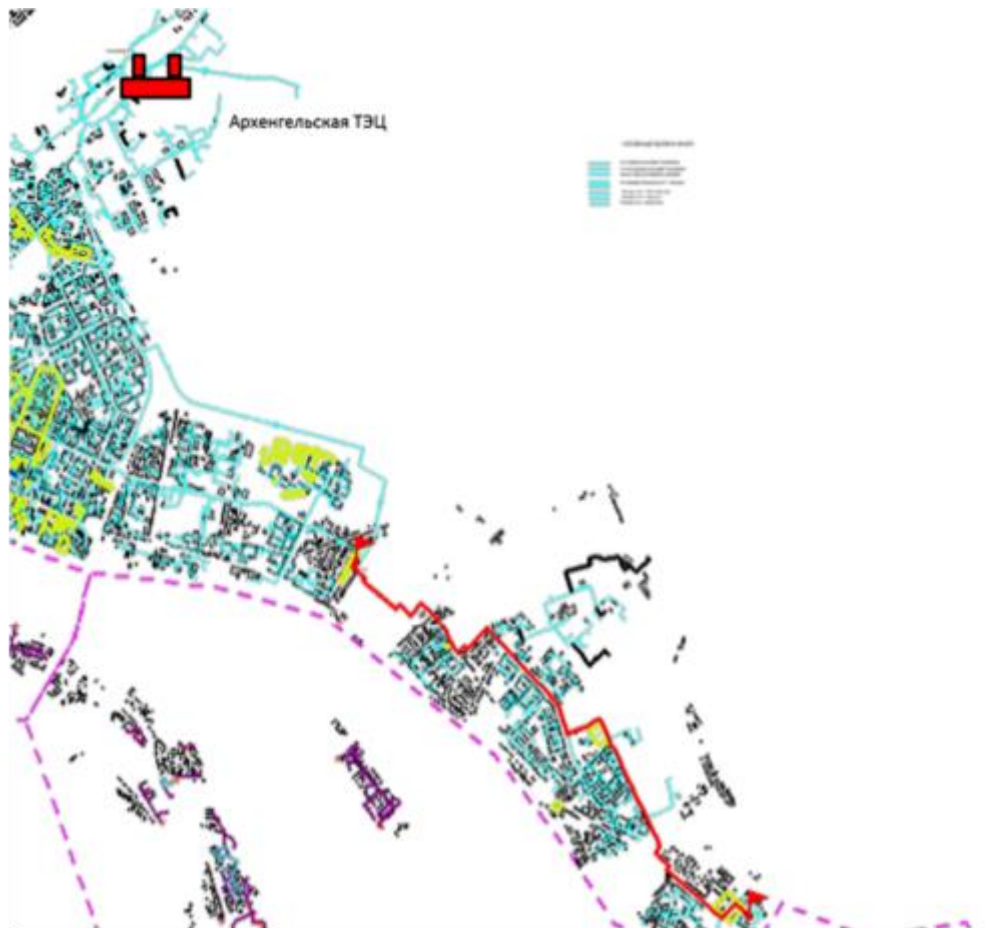
Рисунок 1.4 Путь для расчёта вероятности безотказной работы тепловых сетей от 55-7а до 55-19-16-2
