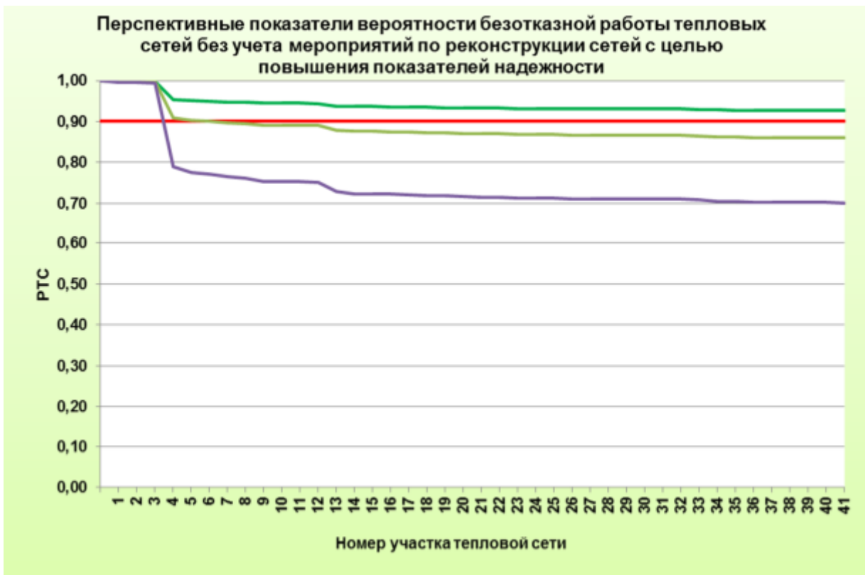
Рисунок 1.5 Вероятность безотказной работы тепловых сетей от 55-7а до 55-19-16-2
