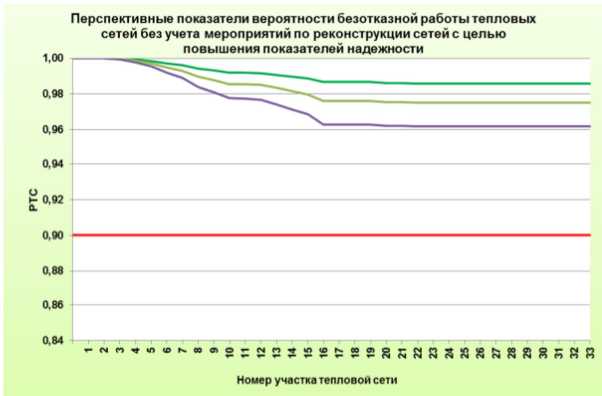
Рисунок 1.8 Вероятность безотказной работы тепловых сетей от Архангельской ТЭЦ до ТК-18г-4
